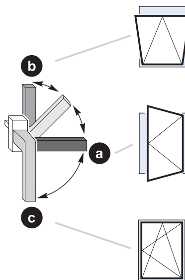
Drehkippenfenster
